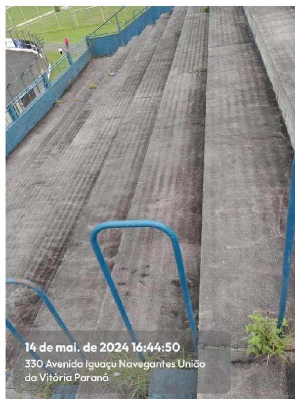
Imagem 53: Infiltração, vegetação intrusiva e desgaste excessivo do concreto em lajes no Setor C
