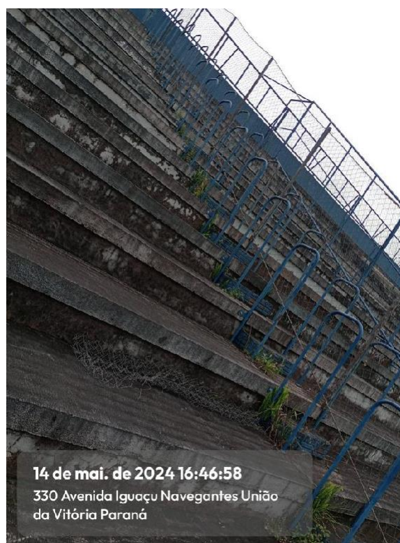
Imagem 52: Infiltração, vegetação intrusiva e desgaste excessivo do concreto em lajes no Setor C
