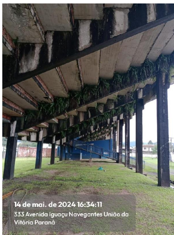
Imagem 64: Infiltração e vegetação intrusiva em vigas, pilares e lajes no Setor D
