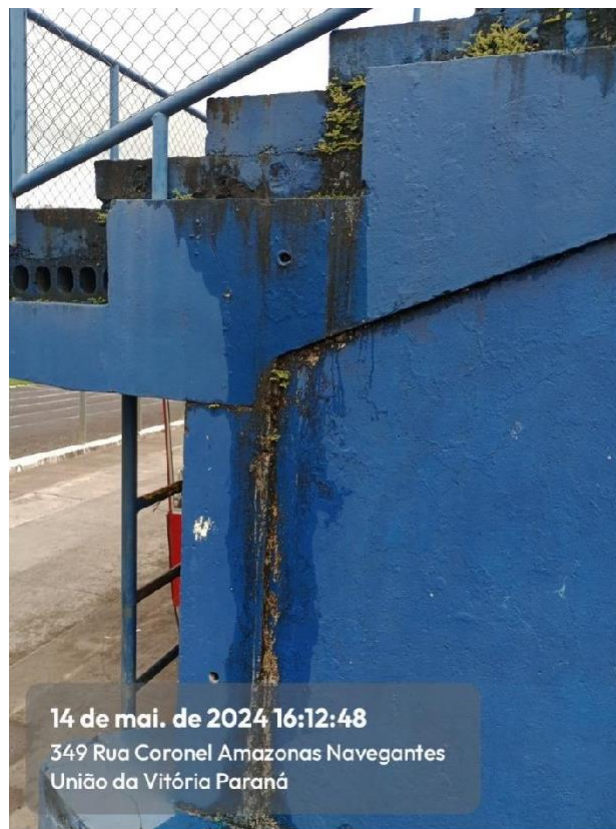
Imagem 02: Infiltração e vegetação intrusiva em lajes, pilar e alvenaria no Setor A
