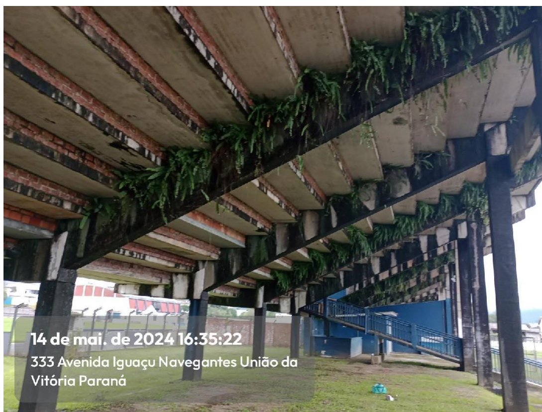
Imagem 69: Infiltração e vegetação intrusiva em vigas, pilares e lajes no Setor D
