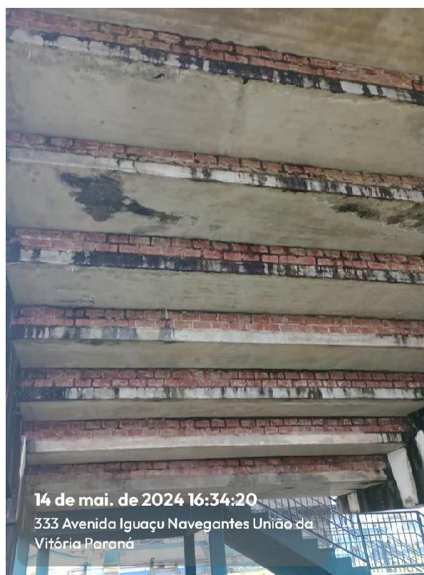
Imagem 65: Infiltração e vegetação intrusiva em vigas e lajes no Setor D
