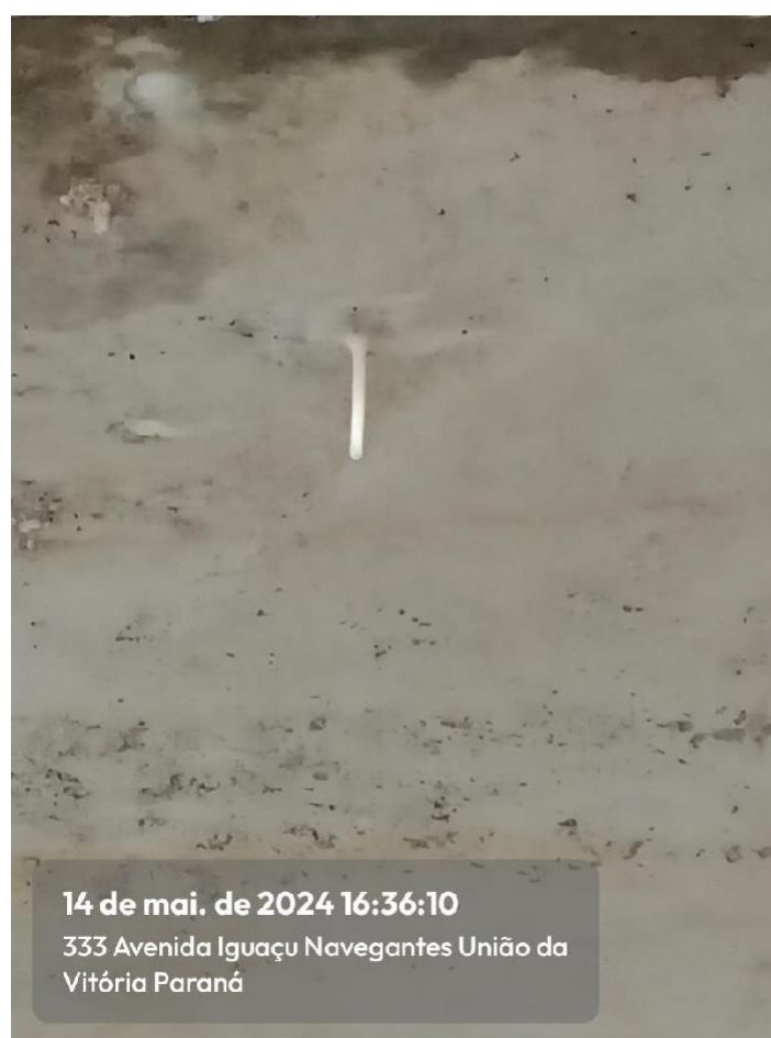
Imagem 72: Infiltração em lajes, com presença de estalactite no Setor D
