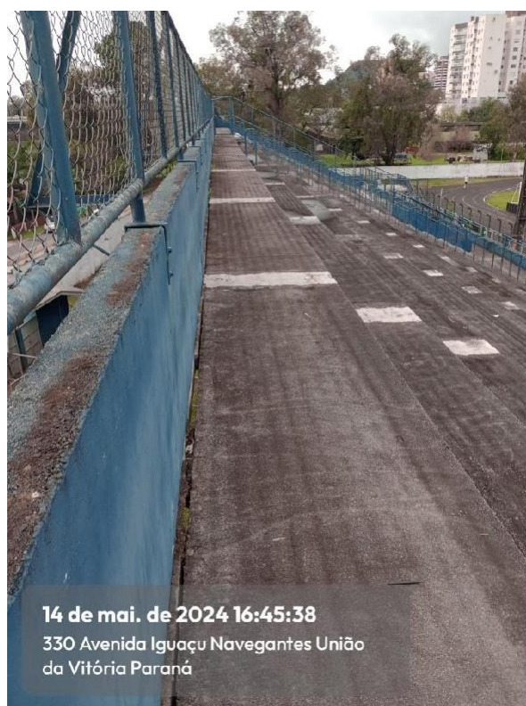
Imagem 55: Infiltração e desgaste excessivo do concreto em lajes no Setor C
