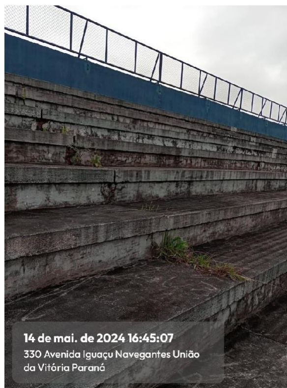
Imagem 51: Infiltração, trincas e vegetação intrusiva em lajes e alvenaria no Setor C
