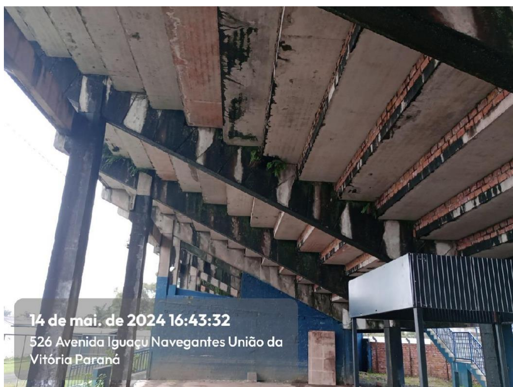
Imagem 46: Infiltração e vegetação intrusiva em lajes, vigas e pilares no Setor C
