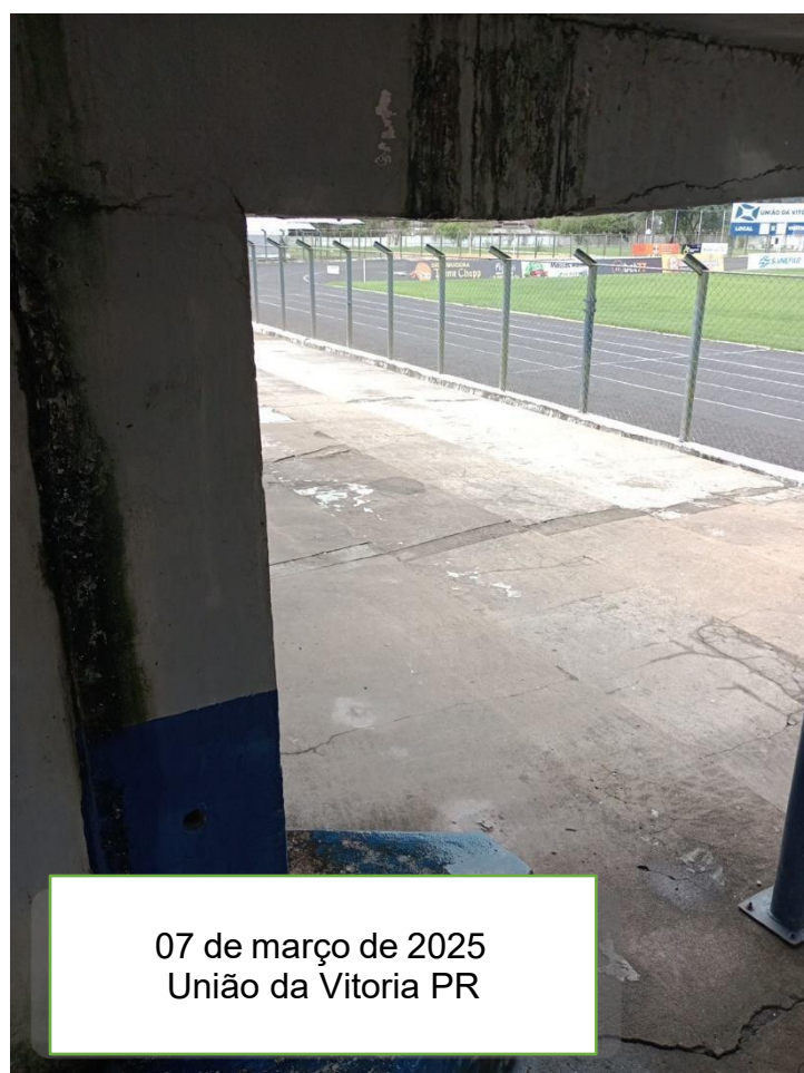
Imagem 31: Infiltração, trincas e vegetação intrusiva em pilar e viga no Setor Cadeiras
