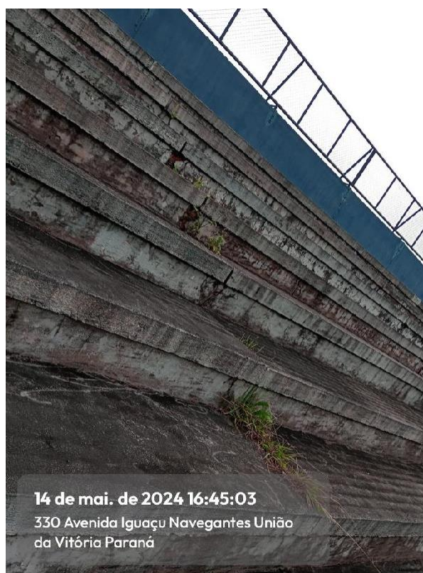
Imagem 50: Infiltração, trincas e vegetação intrusiva em lajes e alvenaria no Setor C
