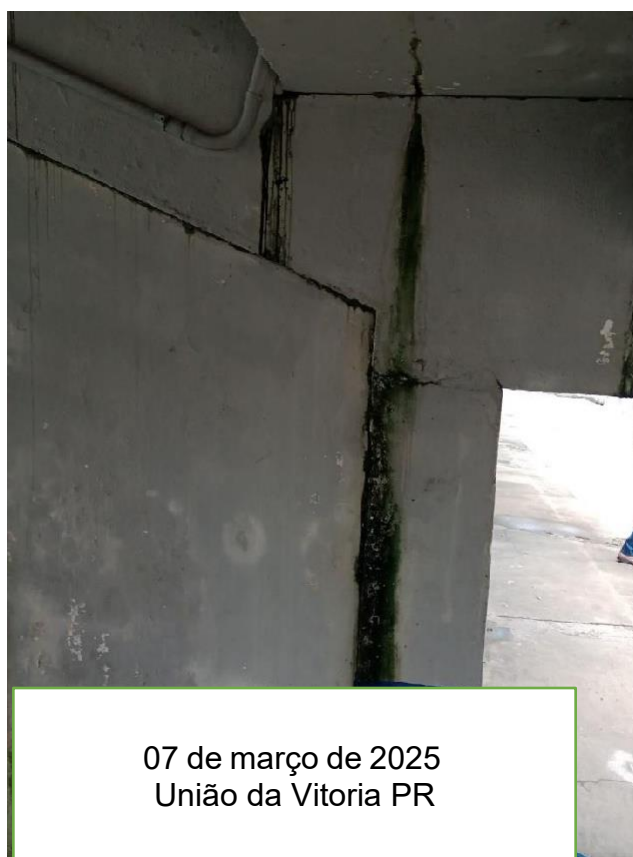
Imagem 10: Infiltração em laje no Setor A
