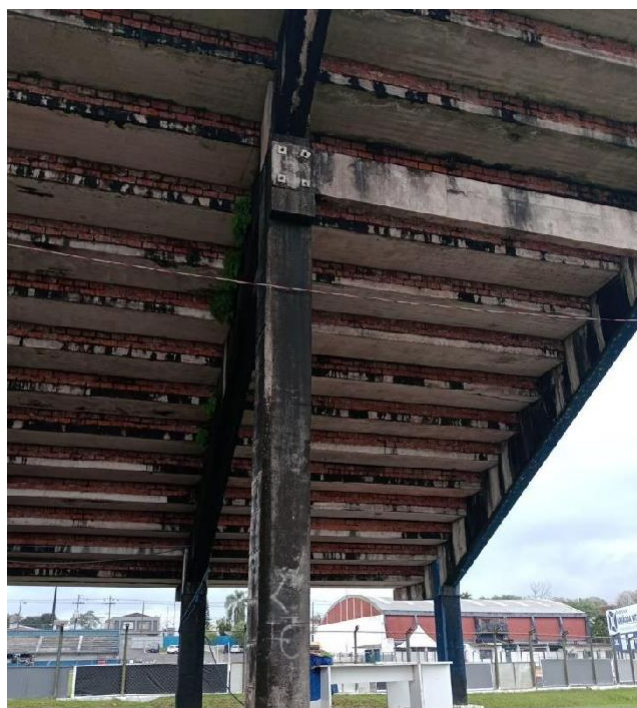
Imagem 43: Infiltração e vegetação intrusiva em lajes, vigas e pilares no Setor C
