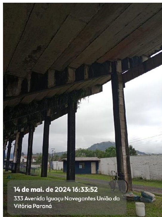
Imagem 63: Infiltração e vegetação intrusiva em vigas, pilares e lajes no Setor D
