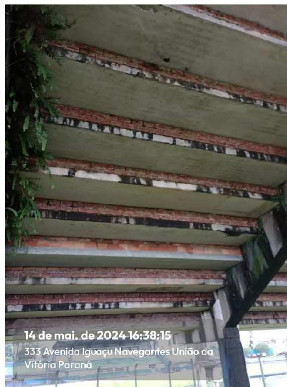
Imagem 74: Infiltração e vegetação intrusiva em vigas, pilares e lajes no Setor D
