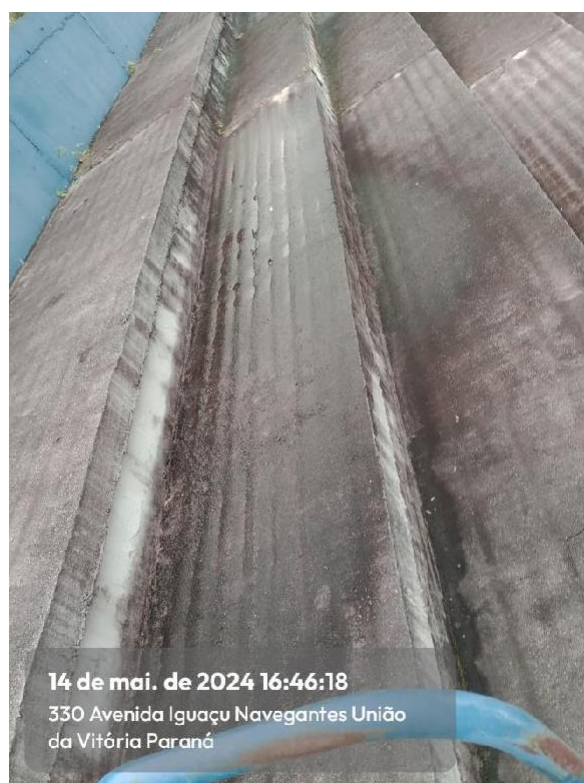
Imagem 57: Infiltração, água empoeada e desgaste excessivo do concreto em lajes no Setor C
